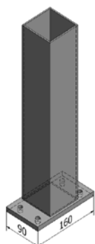
Dübelplatte Zwischenstufe
